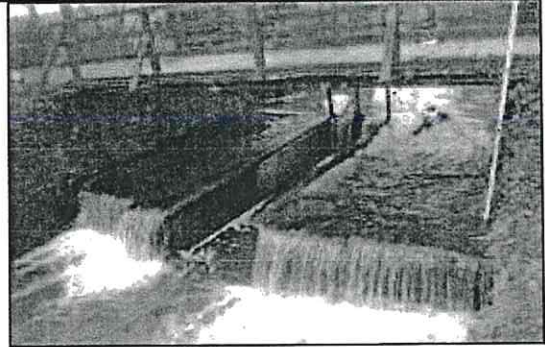
Deux seuils et la vanne (vue aval)
