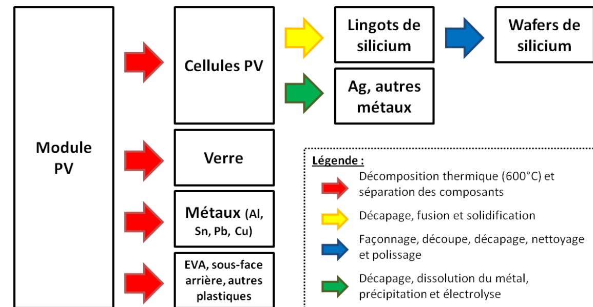
Figure 119 : Processus de recyclage des modules
